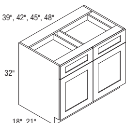
VB3932_ _-VB4832_ _CS Center mullion
